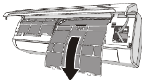
Воздушный фильтр грубой очистки
